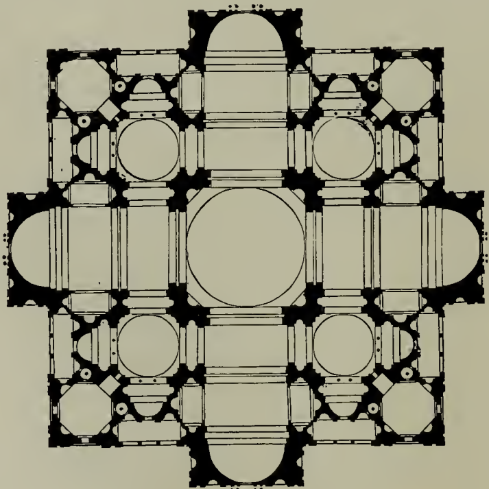
Abb. 104. St. Peter. Bramantes erster Grundriß.
